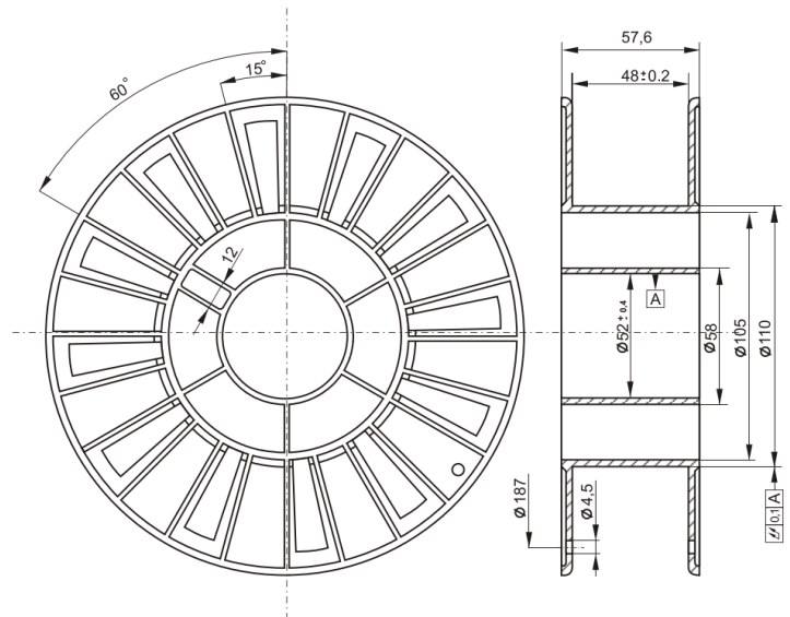
Катушка D200
