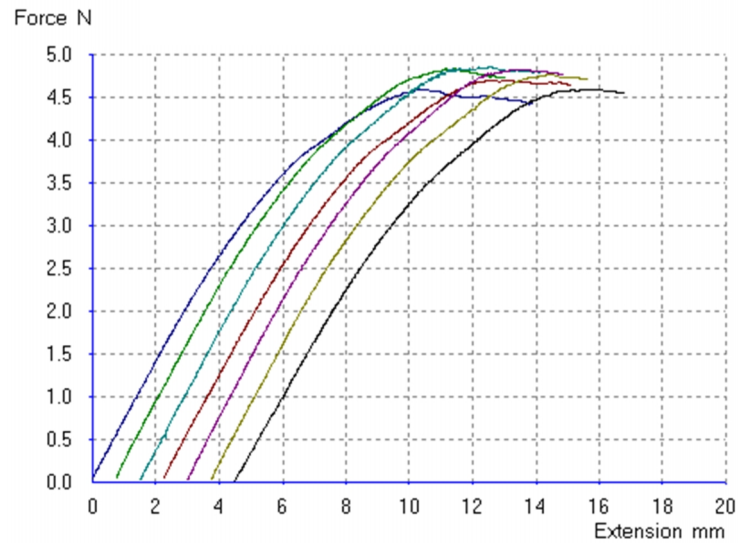
Рис. 1. Зависимость нагрузки от перемещения для образцов 1÷7
