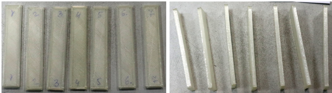
Фотографии элементарных образцов 1÷7 после испытаний
